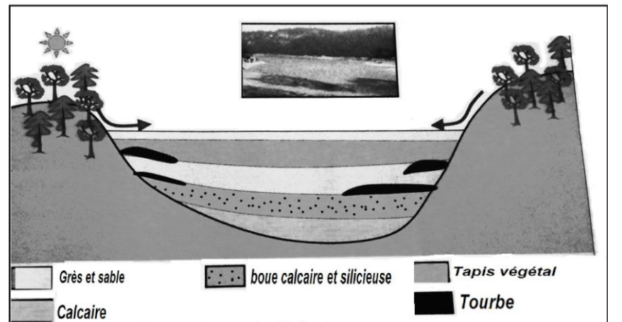
Document 3 : Les types de dépôts lacustres
